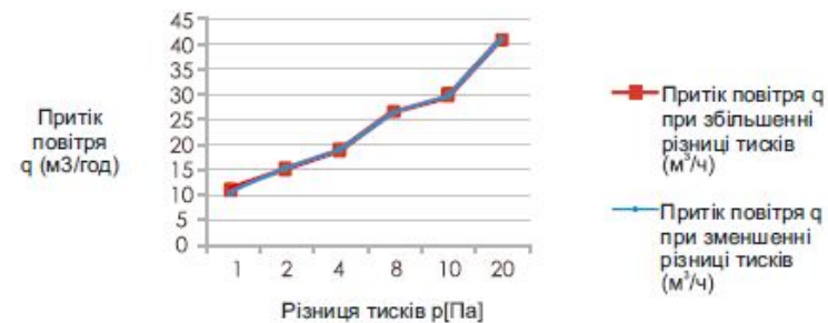
Графік 3. Залежність притоку повітря q (м 3 /год), перетікаючого через провітрювач VT 501, від різниці тисків p (Па)
