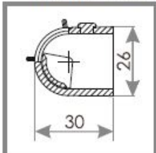
РОЗРІЗ OZ 100
