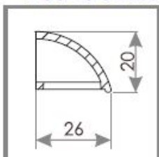
РОЗРІЗ OZ 300
