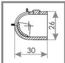
РОЗРІЗ OZ 200
