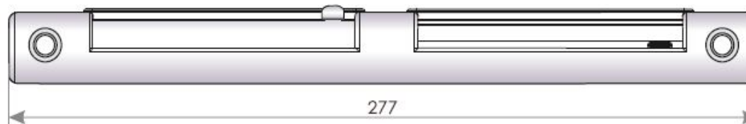
ЗОВНІШНІЙ КЛАПАН OZ 200
