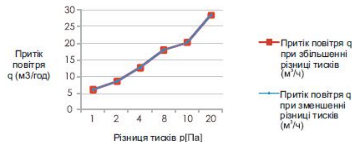
Графік 4. Залежність притоку повітря q ( \text{м}^3/\text{год} ), перетікаючого через провітрювач VT 601, від різниці тисків p (Па)
