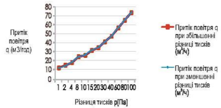
Графік 1. Залежність притоку повітря q ( \text{м}^3/\text{год} ), перетікаючого через провітрювач VT 101, від різниці тисків p (Па)
