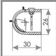
РОЗРІЗ OZ 200
