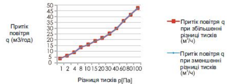
Графік 2. Залежність притоку повітря q ( \text{м}^3/\text{год} ), перетікаючого через провітрювач VT 201, від різниці тисків p (Па)
