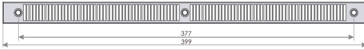
ЗОВНІШНІЙ КЛАПАН ПІД РОЛОКАСЕТИ OZ 300
