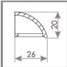
РОЗРІЗ OZ 300
