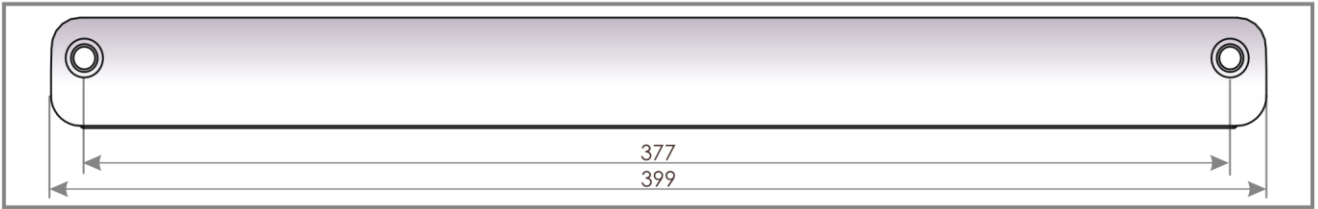
АКУСТИЧНИЙ ЗОВНІШНІЙ КЛАПАН OZ 400
