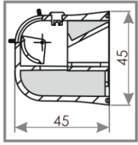
РОЗРІЗ VT 400
