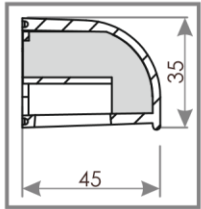
РОЗРІЗ OZ 400
