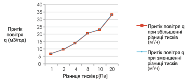
Графік 6. Залежність притоку повітря q (м 3 /год), перетікаючого через провітрювач VT 401, від різниці тисків p (Па)
